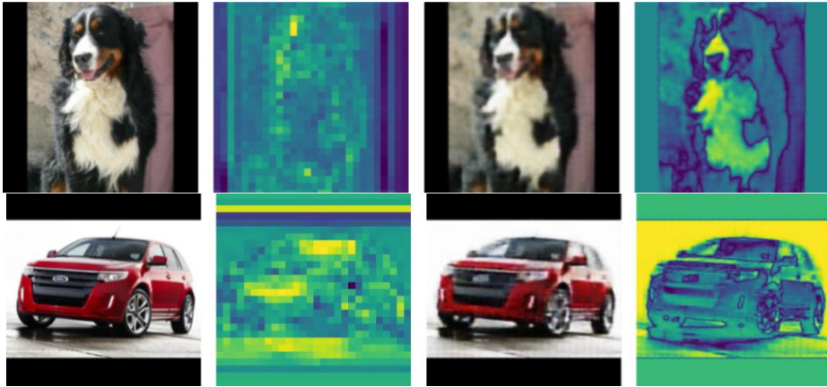
شکل ۵: بازنمایی تصاویر تنک در مدل SAE. به ترتیب از چپ به راست: تصاویر طبیعی، فعال‌ساز ویژگی-های تنک در خروجی انکدر، تصویر بازسازی شده در دیکدر و فعال‌ساز خروجی دیکدر
