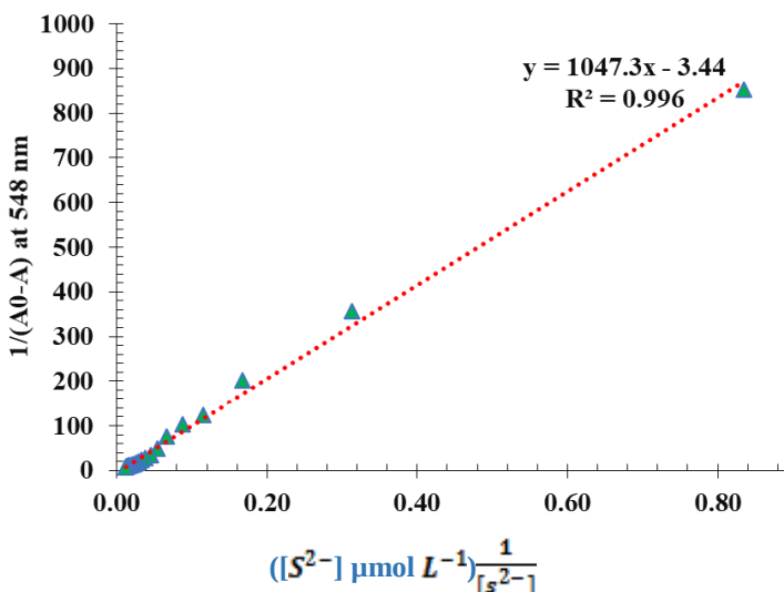
شکل ۶. رسم نمودار 1/(A_0 - A) بر حسب [S^{2-}] ؛ جذب در طول موج ۵۴۸ نانومتر
