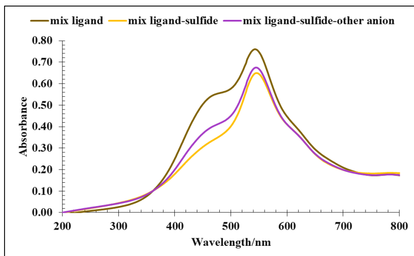
شکل ۷ نمودار گیرنده EBT-Zn 2+ -ERS با افزایش سولفید به همراه سایر آنیون ها (کربنات، بی کربنات، فلورید، اگزالات، برمید، نیترات، سیترات، مونوفسفات، دیدید، کلرید، تیوسولفات و تیوسیانات)
