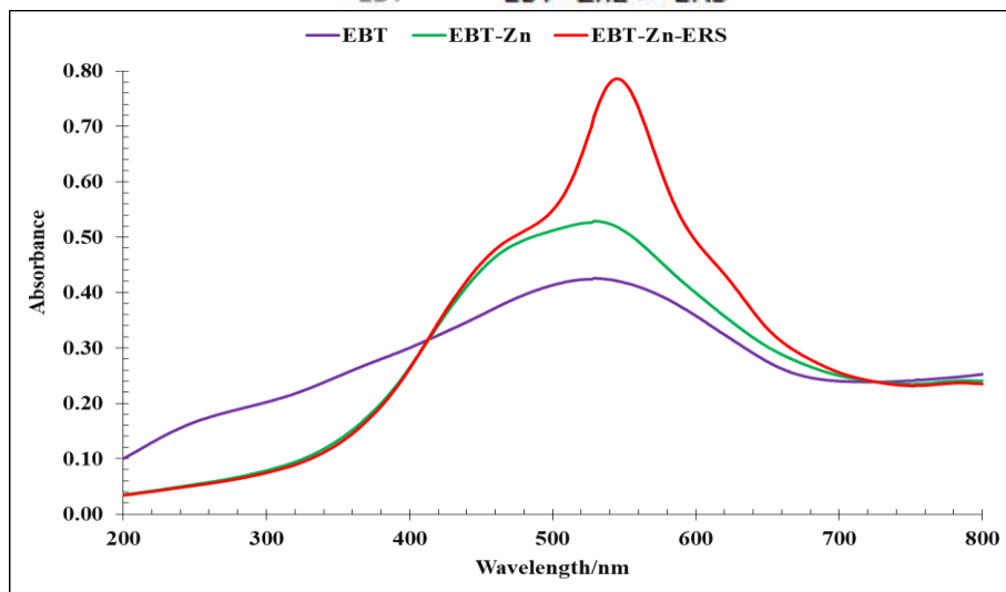
شکل ۲ تغییرات رنگ و طیف جذبی مربوط به EBT، EBT و Zn^{2+} و 1.0 \times 10^{-4} میکرولیتر ERS تشکیل کمپلکس فلزی مخلوط لیگاندها در \lambda_{max} برابر ۵۴۸ نانومتر با جذب ۰/۷۸
