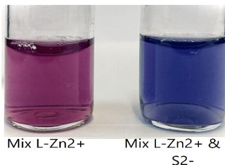
شکل ۴ تغییر رنگ حسگر شیمیایی کمپلکس فلزی مخلوط لیگاندها (EBT-Zn 2+ -ERS) با افزایش ۵۰۰/۰ میکرولیتر (۱۸۵/۰ میکرومولار) از سولفید با غلظت 10^{-3} \times 10^{-1} مولار
