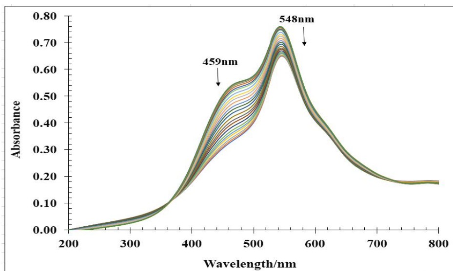
شکل ۳ تغییرات در طیف جذبی UV-Vis کمپلکس فلزی مخلوط لیگاندها (EBT-Zn 2+ -ERS) با افزایش تدریجی سولفید (۰/۰۲-۱۸۵/۰ میکرومولار)
