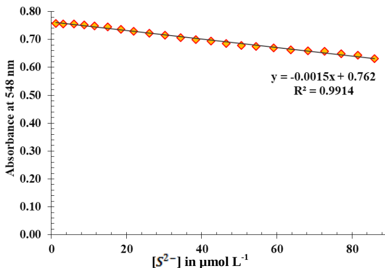
شکل ۹ نمودار کالیبراسیون و محدوده خطی سولفید در طول موج ۵۴۸ نانومتر؛ محدوده‌ی خطی برای سولفید بین ۰/۲۰ تا ۸۵/۹۲ میکرومولار با ضریب همبستگی ( R^2 ) ۰/۹۹۱۴
