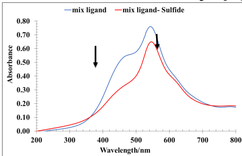
شکل ۵ مقایسه دو طیف کمپلکس فلزی مخلوط لیگاندها (EBT-Zn 2+ -ERS) به همراه ۸۵/۹۲ میکرومولار سولفید؛ کاهش جذب در ۵۴۸ و ۴۵۹ نانومتر
