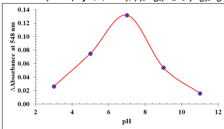
شکل ۸ بهینه سازی pH برای سولفید توسط گیرنده (EBT-Zn 2+ -ERS)؛ این حسگر شیمیایی در pH= ۷/۰ بیشترین میزان تغییرات جذب در شناسایی سولفید
